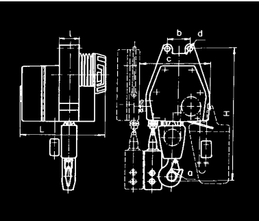
Se závěsným třmenem
