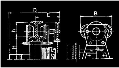
S ručním mechan. vozíkem
