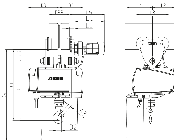
s elektrickým pojezdovým ústrojím EF
