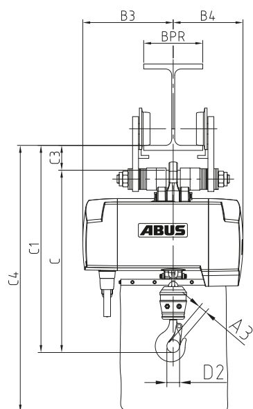
s ručním pojezdovým ústrojím HF
