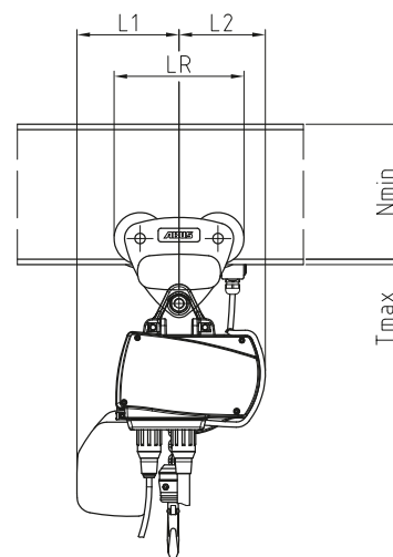
s elektrickým pojízdným ústrojím EF
