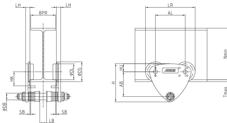
Tabulka rozměrů ručních pojízdoých ústrojí HF firmy ABUS
