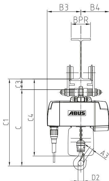
s ručním pojízdným ústrojím HF
