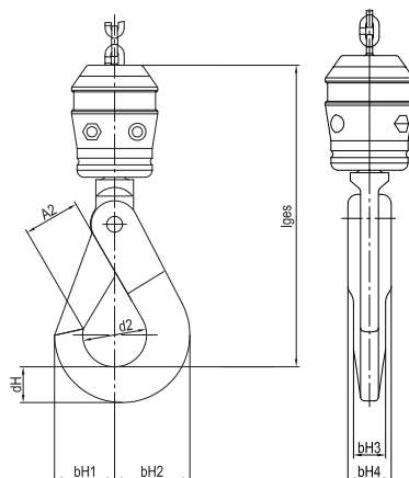
Břemenové hák
