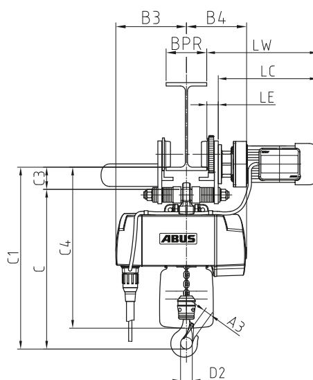
s elektrickým pojízdným ústrojím EF
