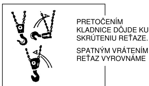
Obr. 2 Pretočenie Reťaze
