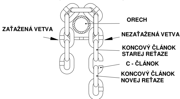
Obr. 11.2 – Výmena bremenovej reťaze
